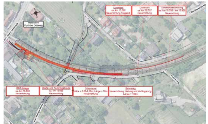
Übersichtslageplan der Baumaßnahmen
